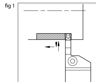
fig 1 Avant le chariotage, reculer l'outil d'environ 0,1 mm après le rainurage (profondeur de rainurage supérieure à 0,5 mm : à l'ébauche).
