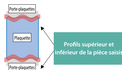
Nouveau système de serrage des plaquettes « W Grip »
